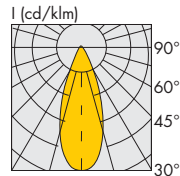
AR111, 12 Вт 60°
