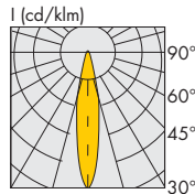
AR111, 12 Вт 38°
