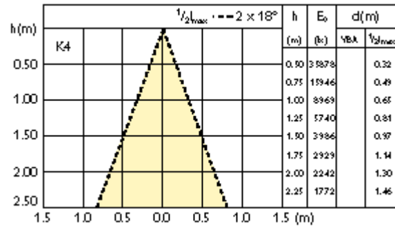
CDM-R111 70W/830 40D
